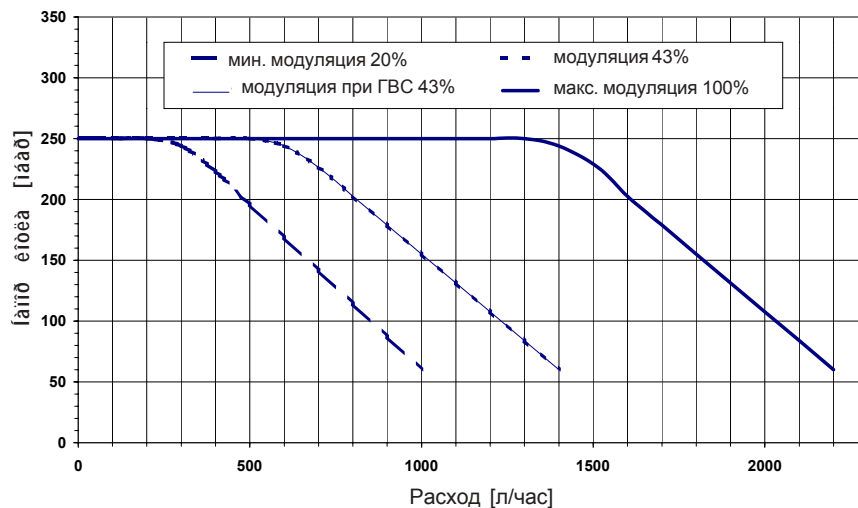
CGB-35 диаграмма насоса с плавной регулировкой числа оборотов
