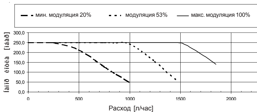
CGB-K40-35 диаграмма насоса с плавной регулировкой числа оборотов
