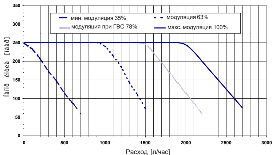
CGB-50 диаграмма насоса с плавной регулировкой числа оборотов
