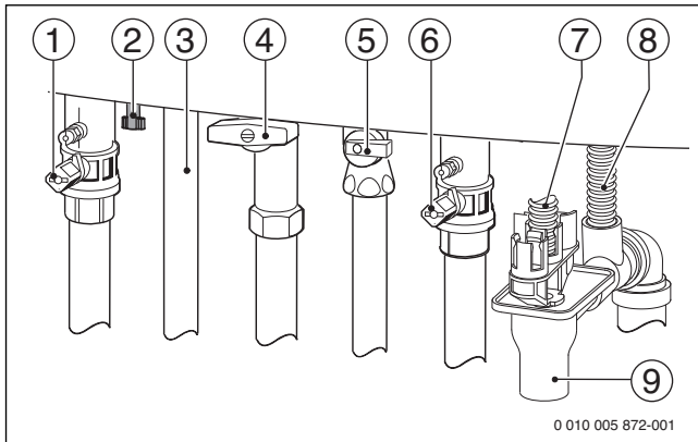
Рис. 1 Подключения газа и воды (дополнительная комплектация)
