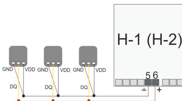
Датчик DS18B20
