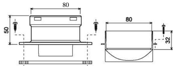
Рисунок 12 – Соединительный элемент для отдельных труб
