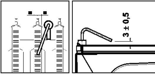
Рисунок 16 – Положение электрода
