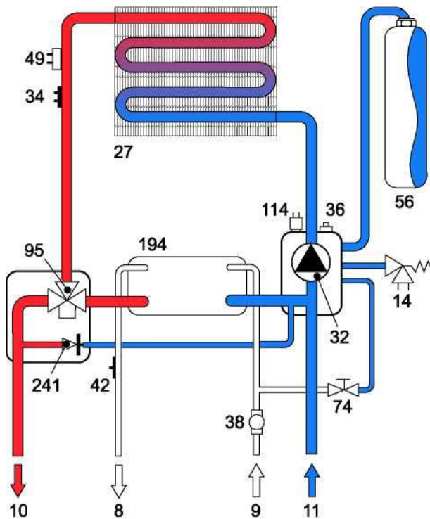
Рисунок 18 – Отопительный контур
