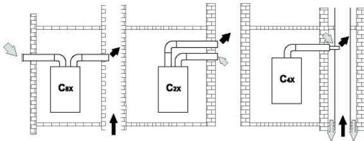
Рисунок 13 – Примеры подсоединения к коллективным дымоходам (светлая стрелка – воздух; темная стрелка – дымовые газы)
