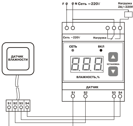
Рис.2 Схема подключения регулятора
